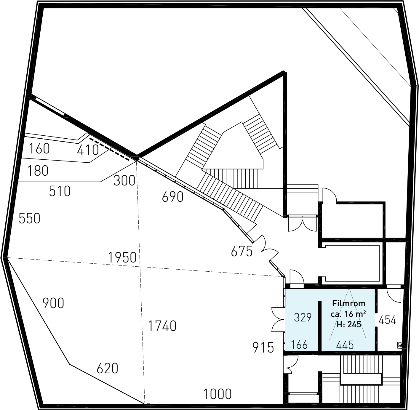
SFKM 4. etasje: Film / Video-rom / Takterrasse. Mål i cm SFKM Third floor: Film / Video-room / Rooftop. Measures in cm
